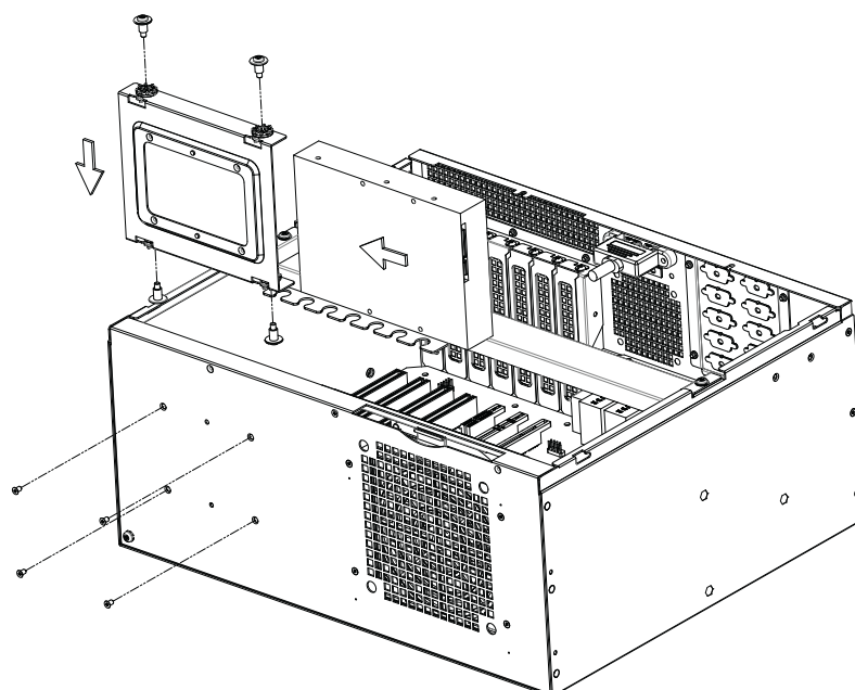
Figure 2.3 Installing internal 3.5" HDD/ 安装内置 3.5" 硬盘 / 安裝內裝 3.5" 硬碟
