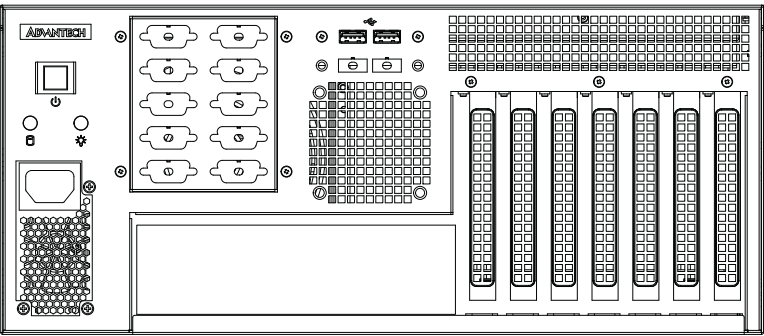
Figure 3.1 Front panel / 前视图 / 前視圖
