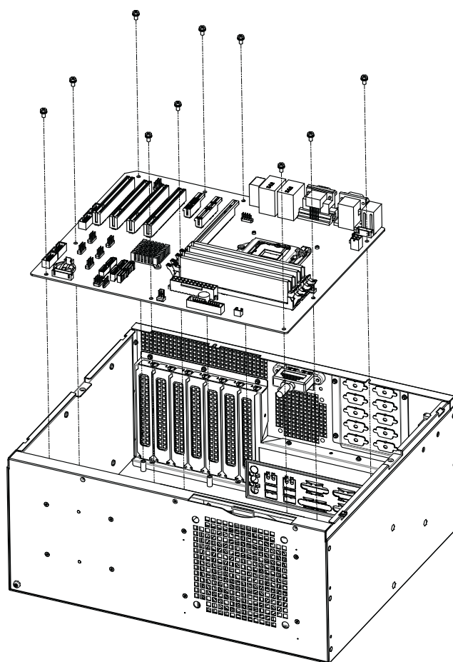
Figure 2.4 Installing a Motherboard/ 安装母板 / 安装主機板
