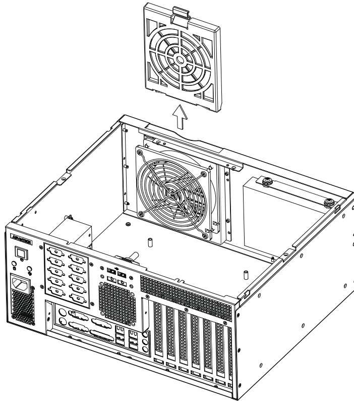
Figure 3.4: Removing the Filters/ 取出过滤器 / 取出濾網
