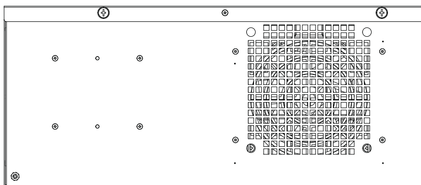
Figure 3.2 Rear panel for motherboard version / 后面板（母板版本） / 後面板（主機板版本）
