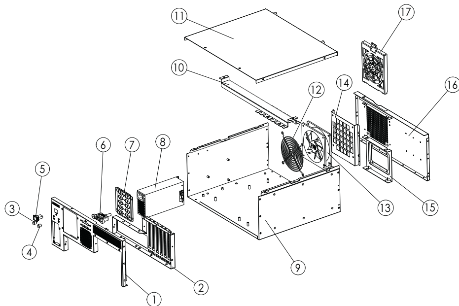
Figure A.1 Exploded Diagrams & Parts List/ 分解图 & 部件列表 / 分解圖 & 零件表
